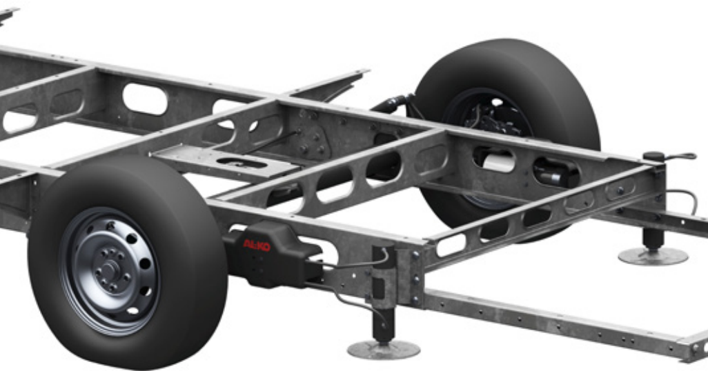
Al-Car: Easynav für den Fiat Ducato
