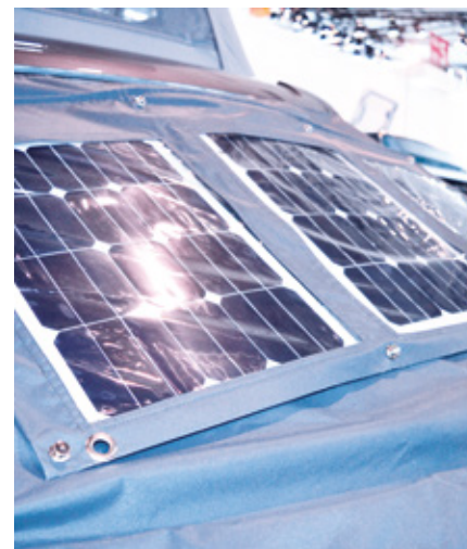
Köhler: Anklipbares Solarpaneel
